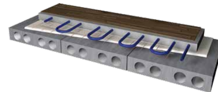
Ontelolaatta / betonipohja
