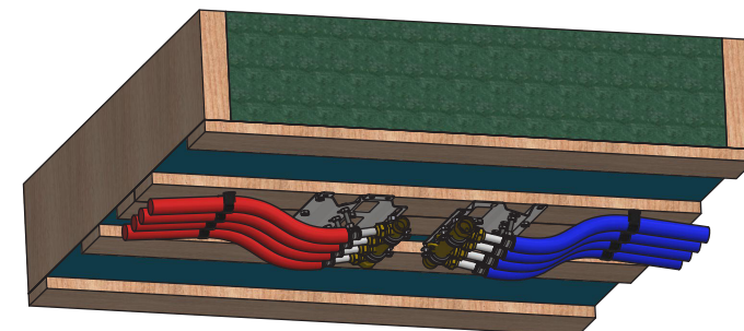
2. VAAKA-ASENNUS
