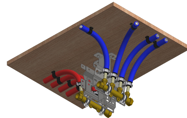
1. PYSTYASENNUS
