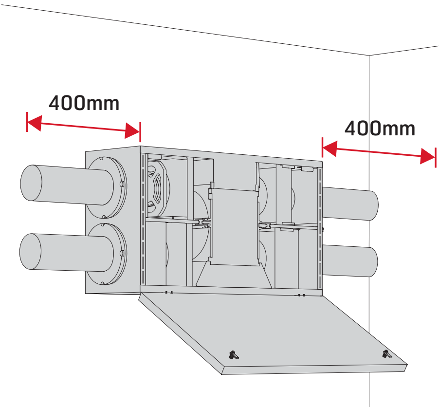
kuva 12 Tilantarve seinäasennuksessa
