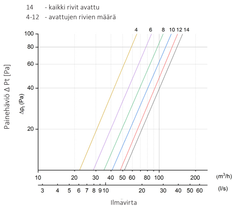
HSTI-125:n painehäviökaavio
