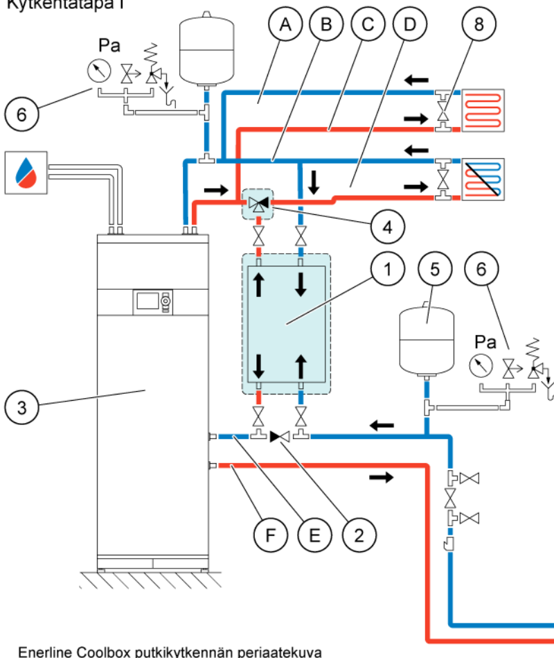
Enerline Coolbox putkikytkennän periaatekuva
