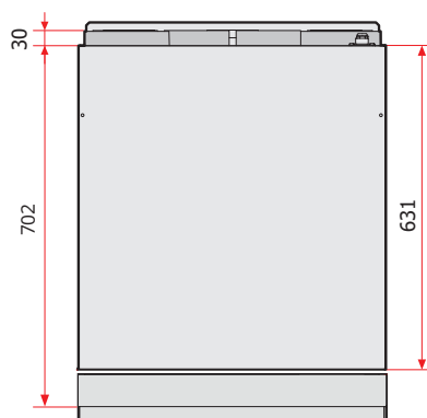
Slimline-liesituuletin lisätarvikkeineen
